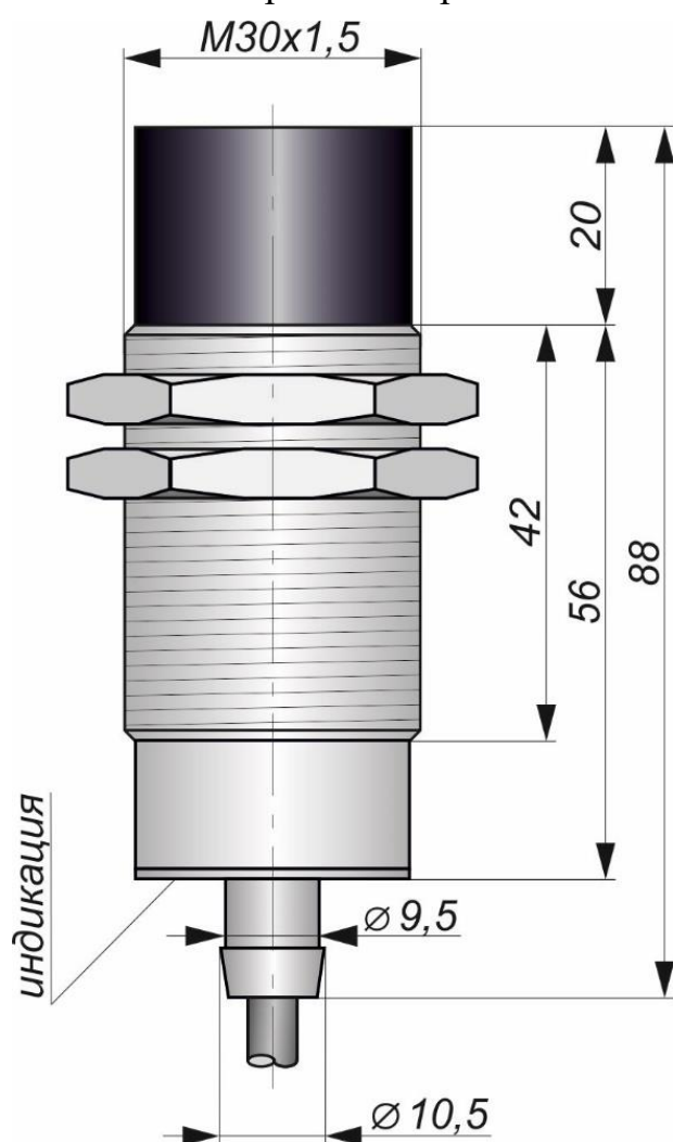
Габаритный чертеж
